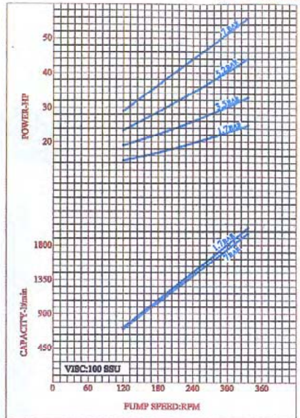
CURVE NO:53AB-02
