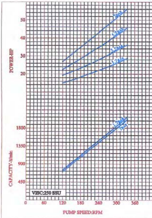
CURVE NO:53AB-03
