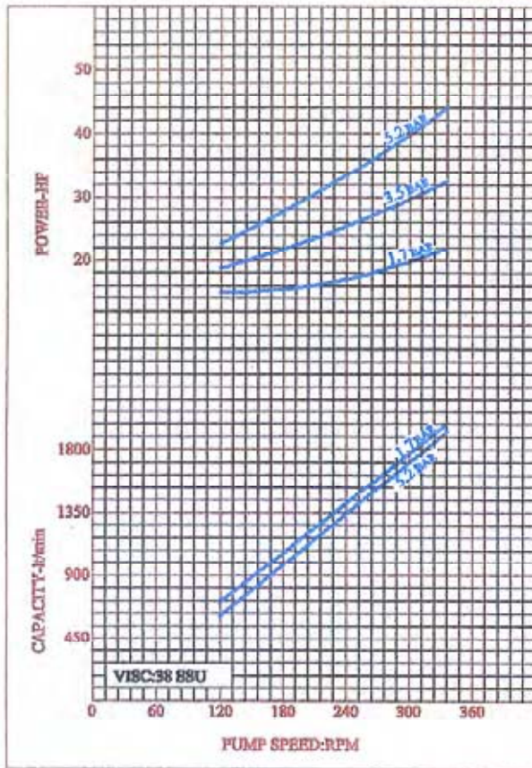
CURVE NO:53AB-01
