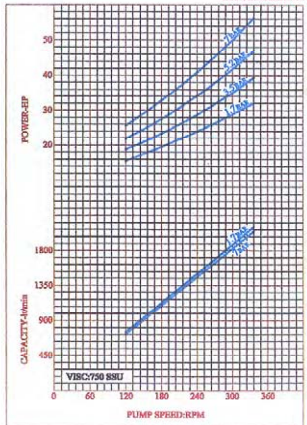
CURVE NO:53AB-04
