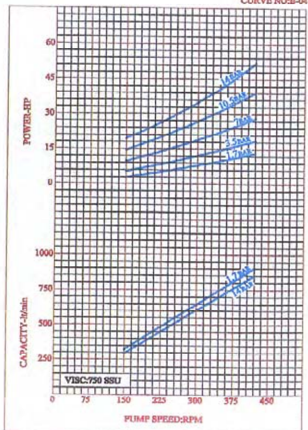
CURVE NO:B-04
