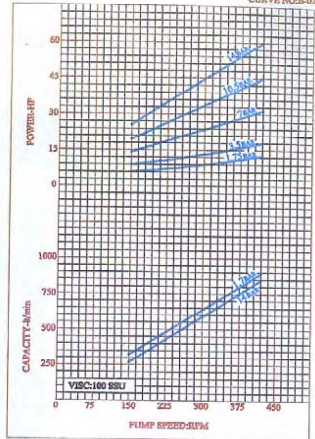
CURVE NO:B-02
