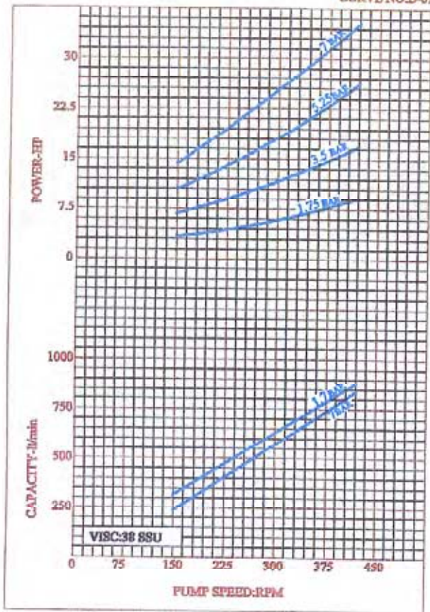
CURVE NO:B-01
