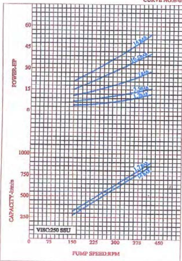
CURVE NO:B-03
