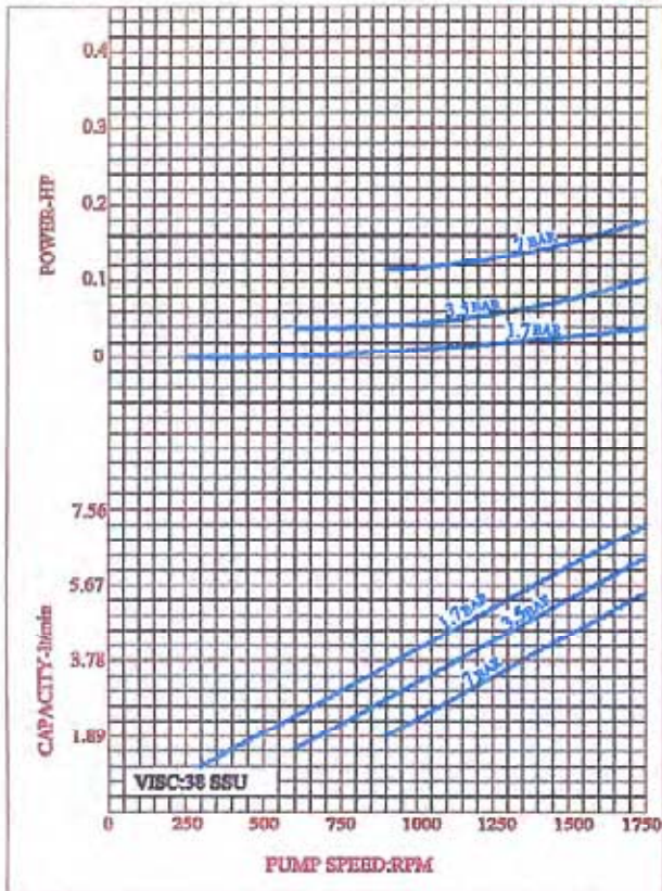
CURVE NO:ME-01
