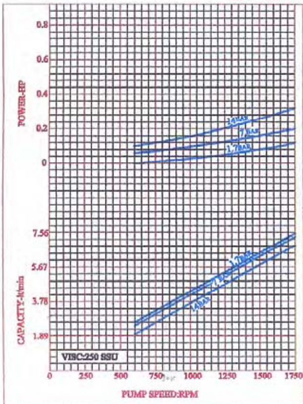
CURVE NO:ME-03
