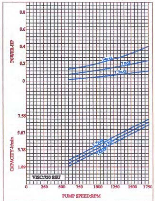
CURVE NO:ME-04
