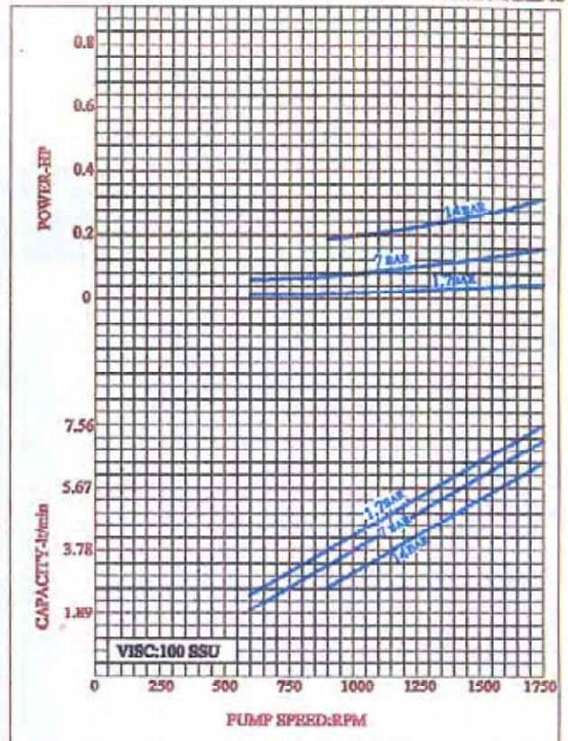
CURVE NO:ME-02
