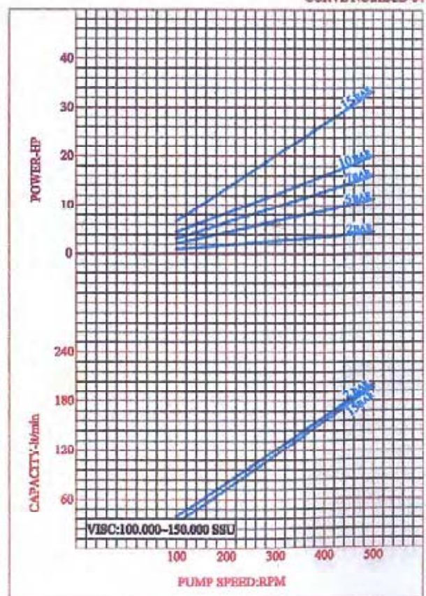
CURVE NO: XLCB-04
