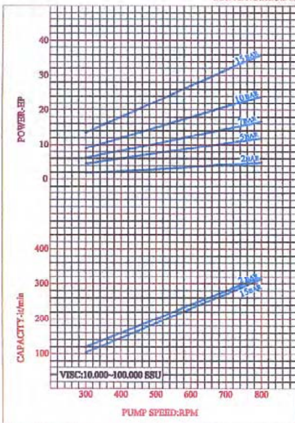
CURVE NO: XLCB-05
