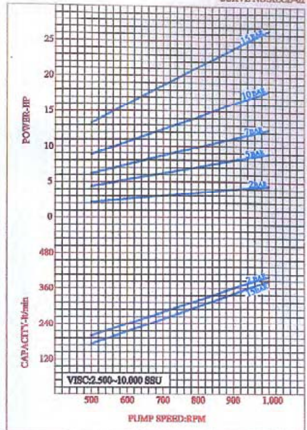
CURVE NO: XLCB-02
