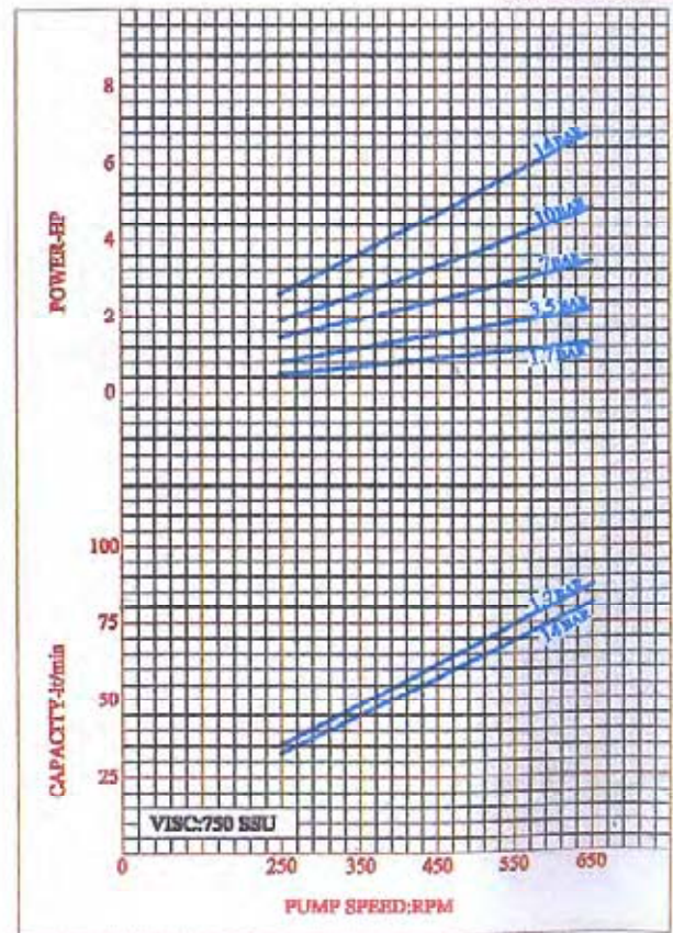
CURVE NO:CDE-04
