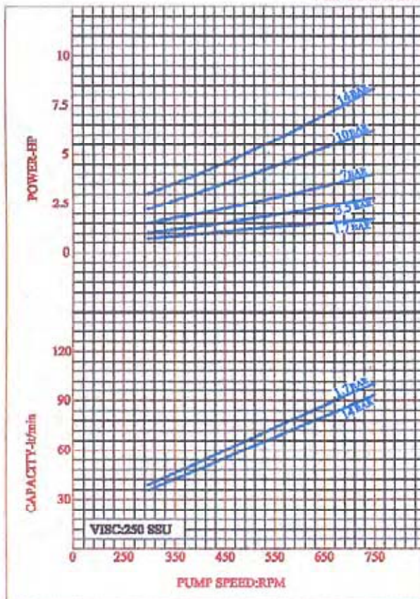
CURVE NO:CDE-03
