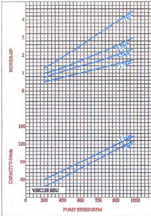
CURVE NO:CDE-01
