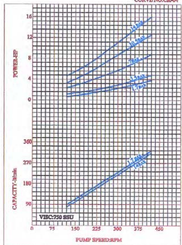
CURVE NO:CK-04
