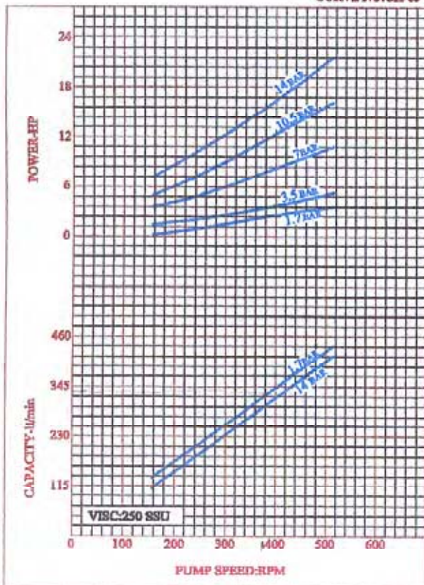
CURVE NO:CK-03
