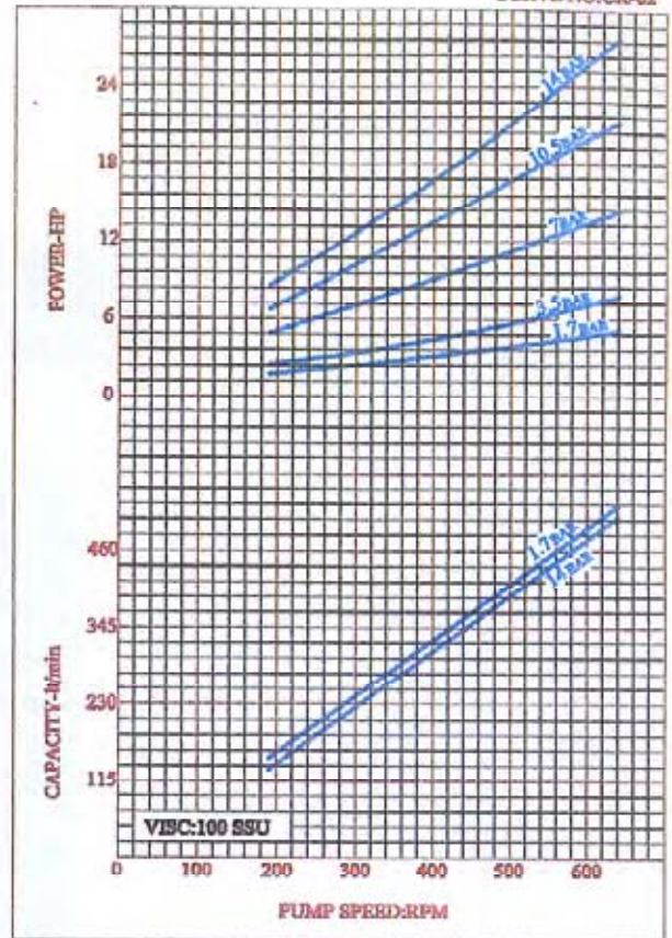
CURVE NO:CK-02
