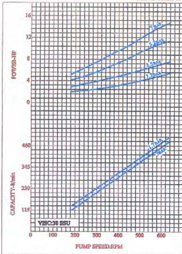
CURVE NO:CK-01
