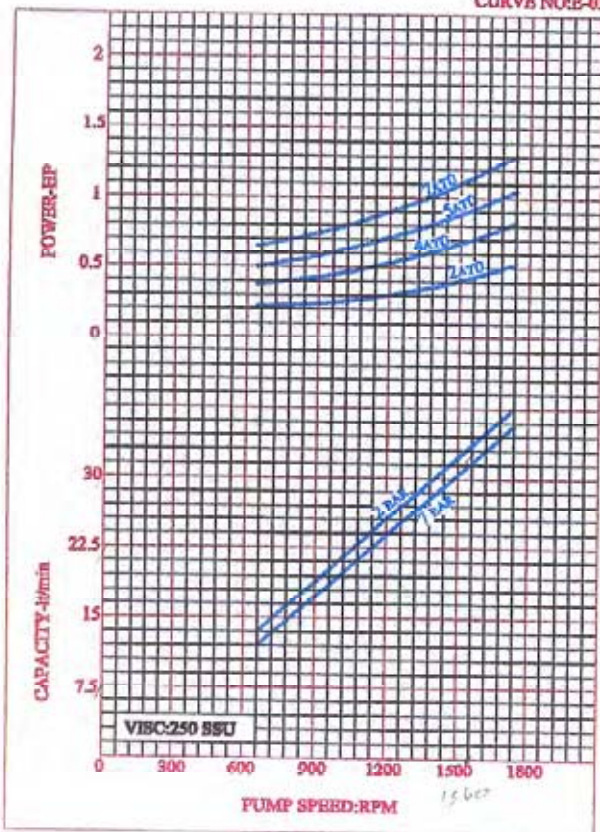
CURVE NO:E-03
