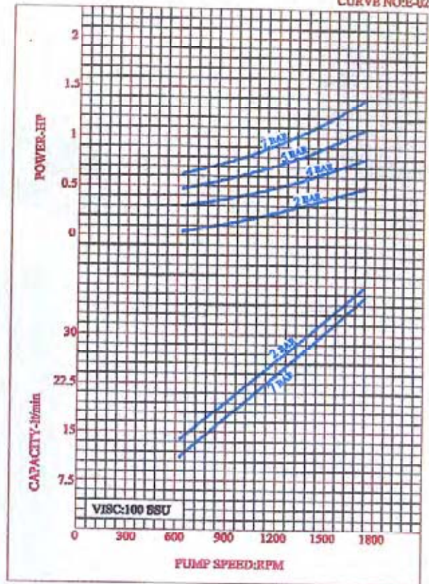
CURVE NO:E-02
