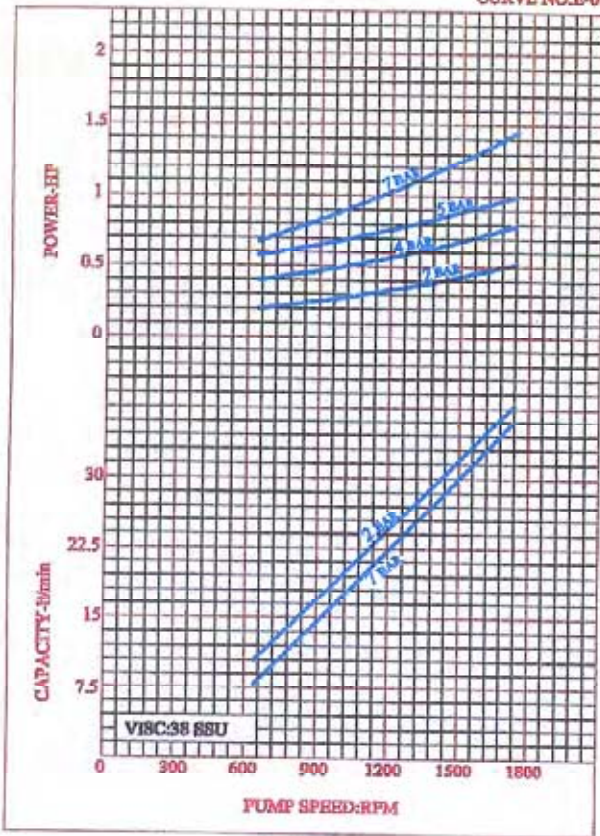
CURVE NO:E-01
