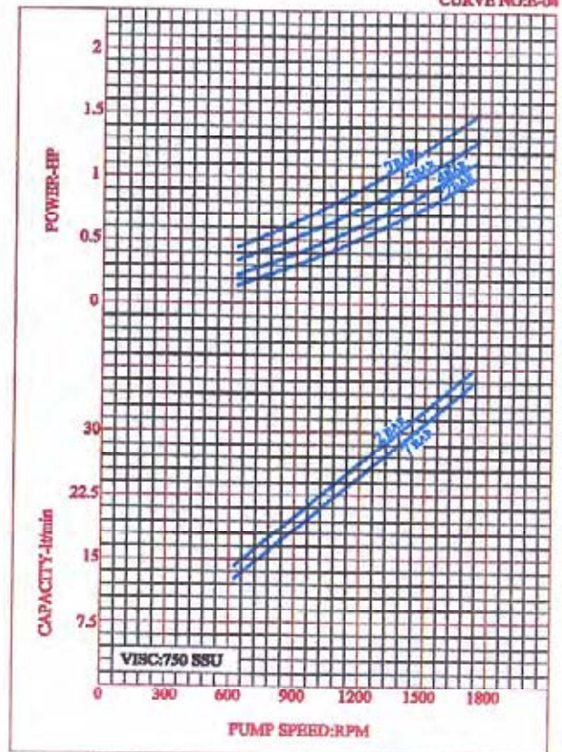
CURVE NO:E-04
