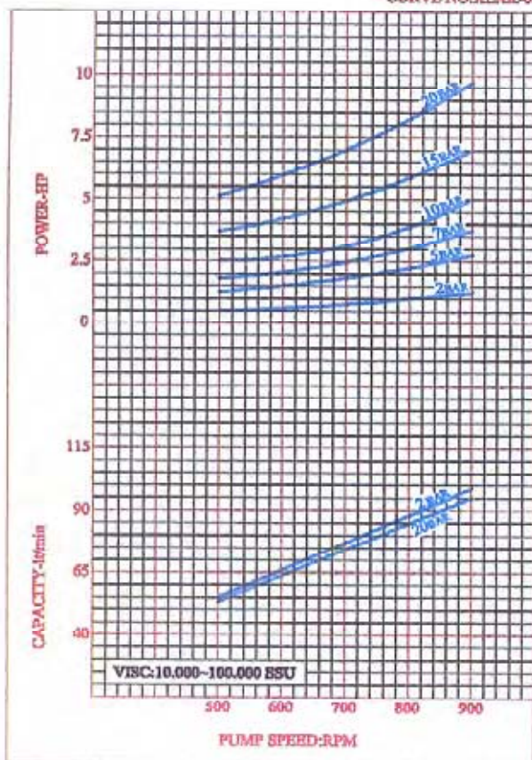
CURVE NO:XLAK-03
