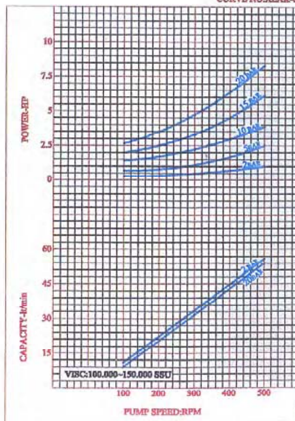
CURVE NO:XLAK-04
