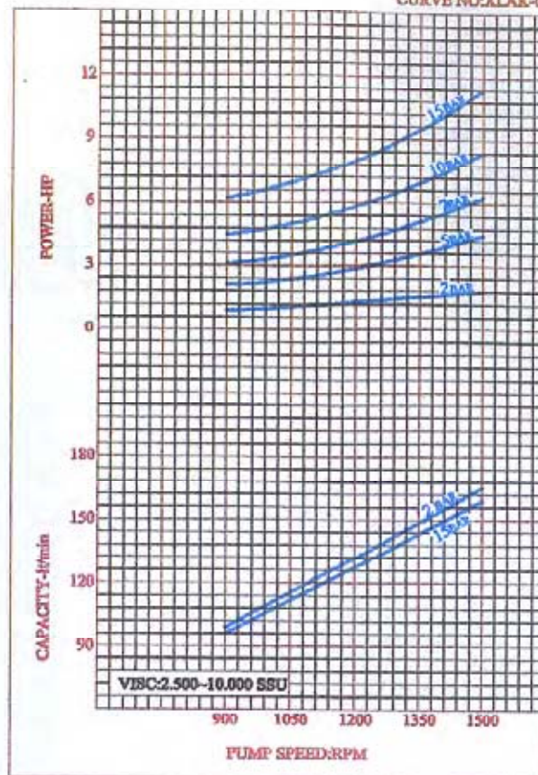
CURVE NO:XLAK-02
