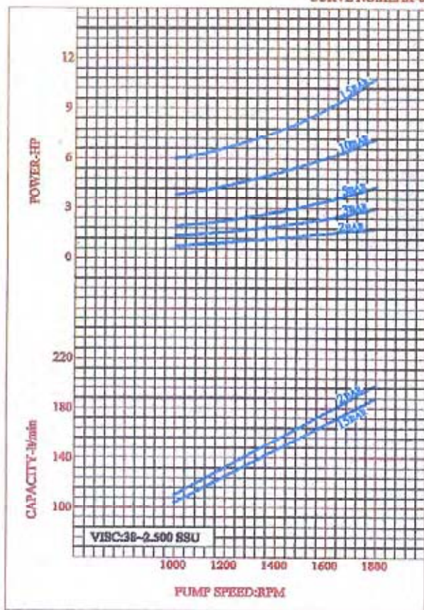
CURVE NO:XLAK-01
