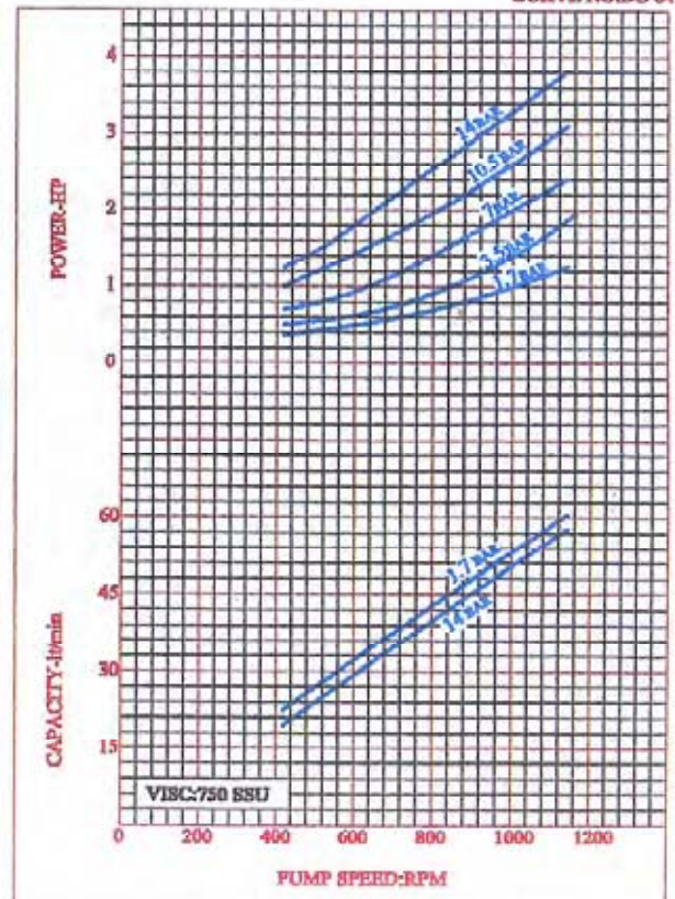
CURVE NO:DC-04
