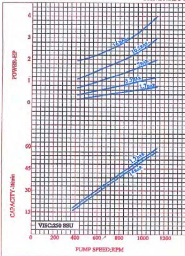
CURVE NO:DC-03
