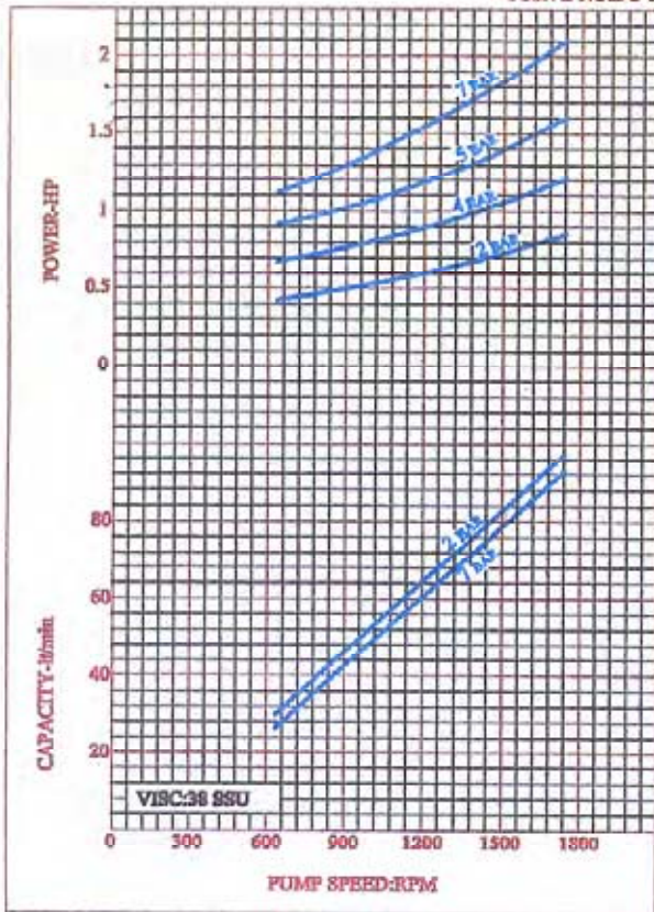
CURVE NO:DC-01
